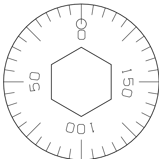
調整ネジ部拡大図 (1目盛0.005)
