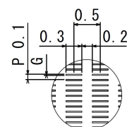
スリット部詳細
