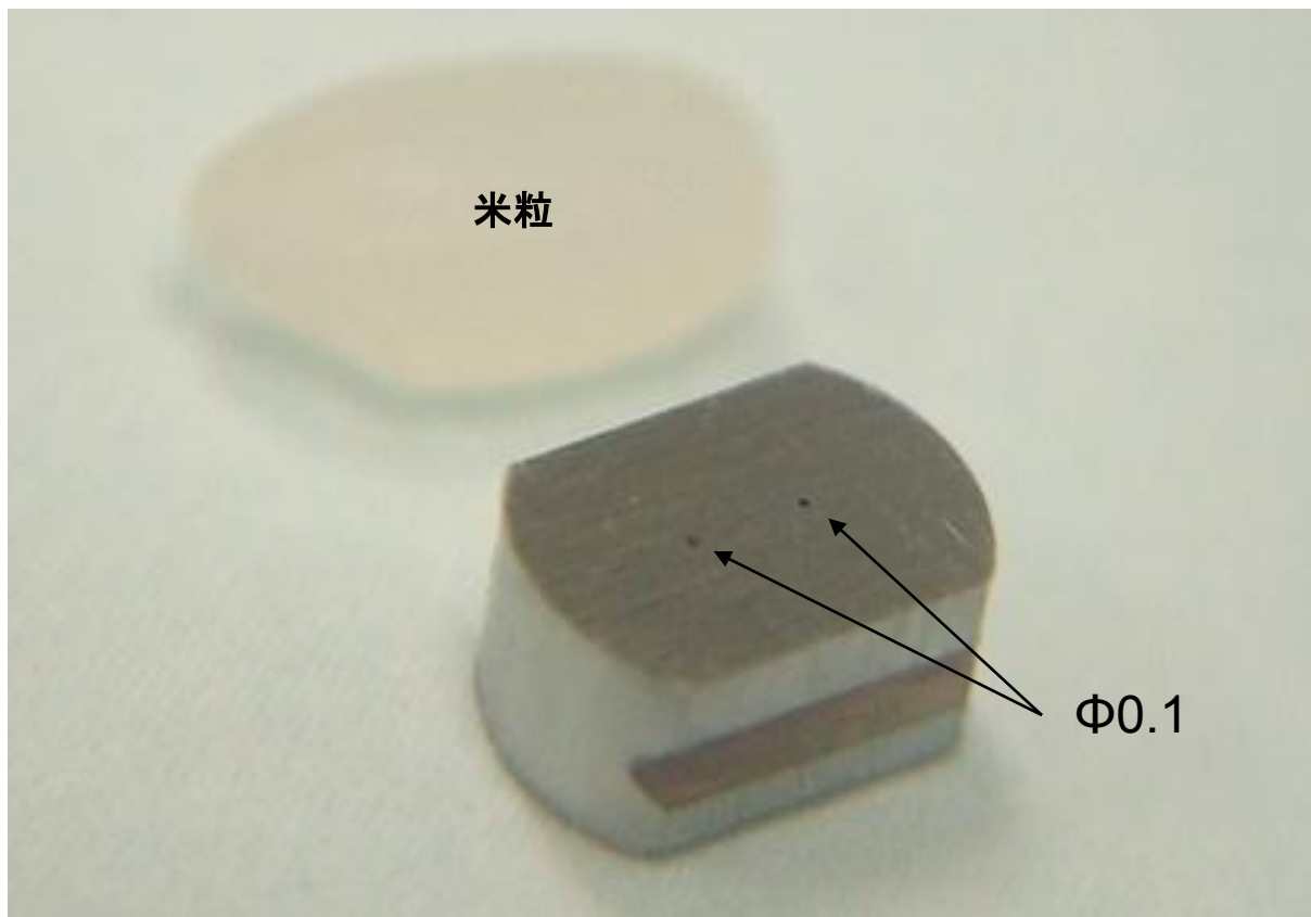
先端部ピースと穴径
