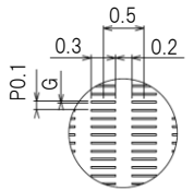
先端詳細図
