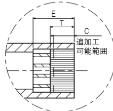
先端スリット部断面
